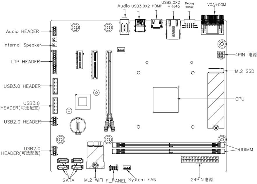
接口位置图
