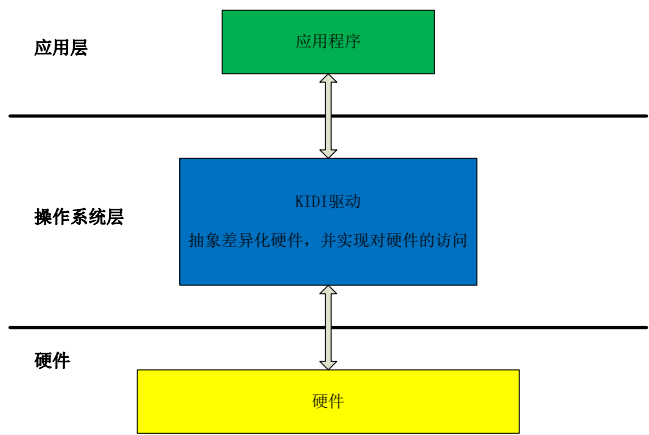
图 5.1 KIDI 架构
