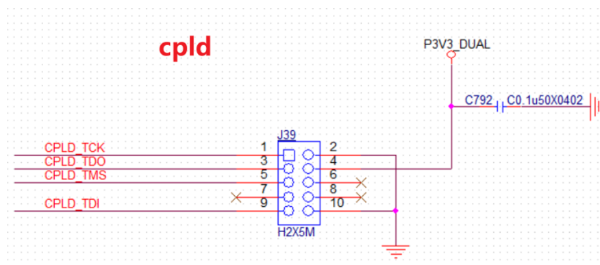
图 2-15 CPLD Header
