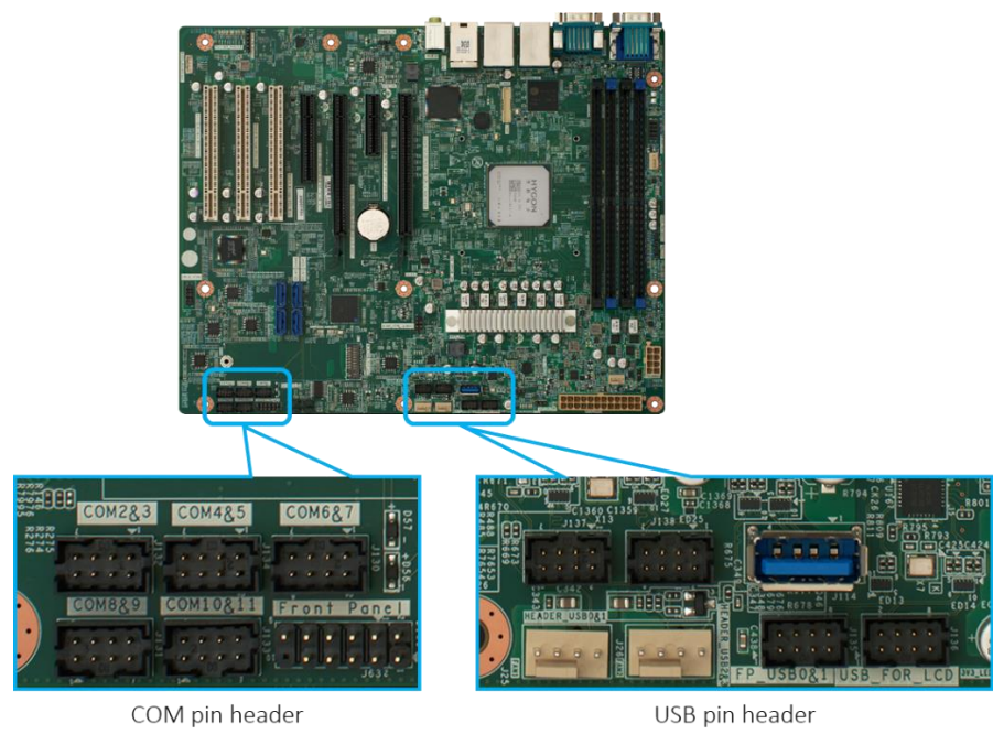
图 2-9 主板 USB/COM 插针位置
