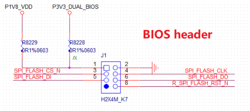
图 2-14 BIOS Header
