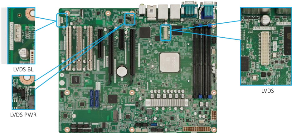
图 2-12 LVDS 插针位置
