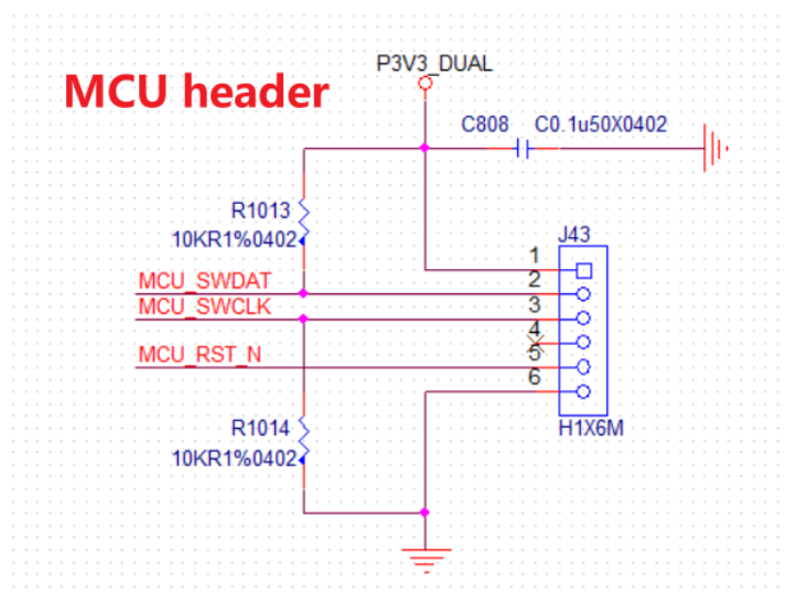
图 2-16 MCU Header
