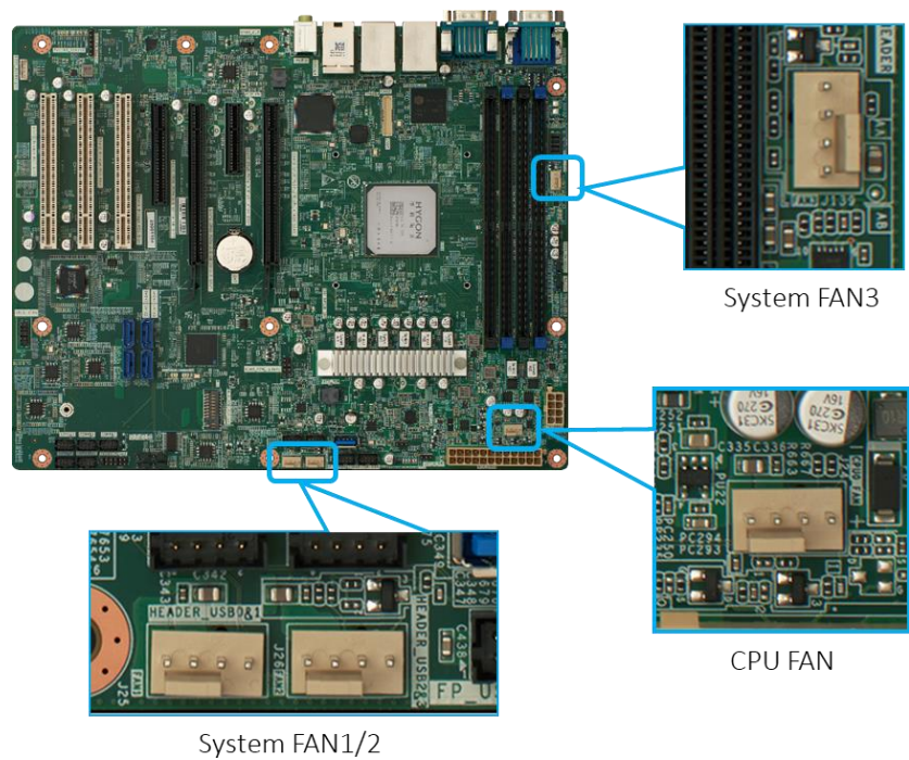
图 2-5 主板散热风扇位置
