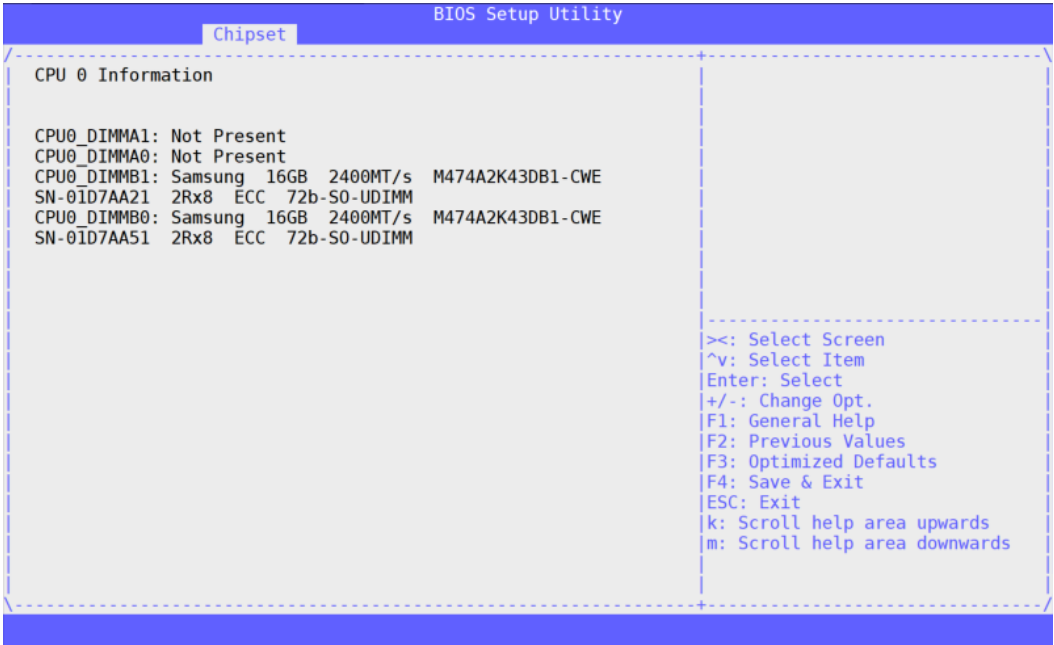
图 3-25 CPU 0 Information
