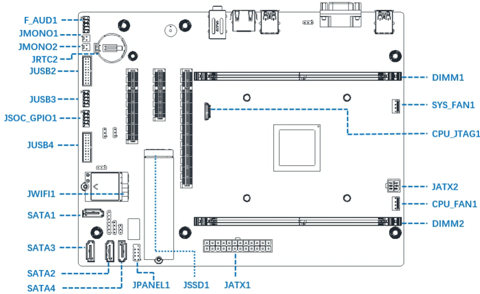
接口位置图
